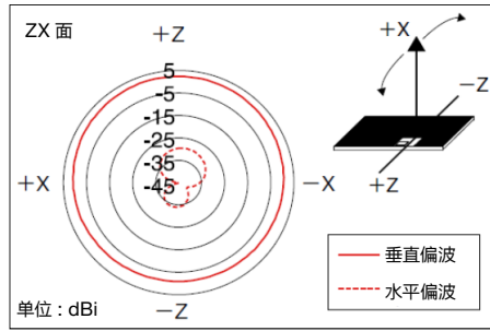
辐射特性代表例 (@1.575GHz)
