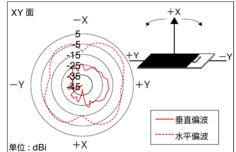
辐射特性代表例 (@5.25GHz)
