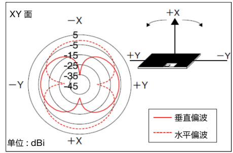
辐射特性代表例 (@1.575GHz)
