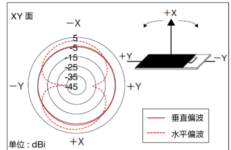
辐射特性代表例 (@3.96GHz)
