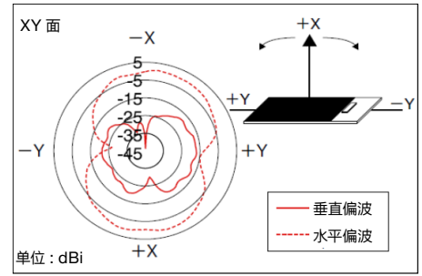
辐射特性代表例 (@2.45GHz)
