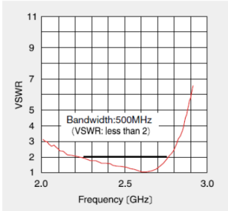
VSWR特性代表例 (2GHz频带)
